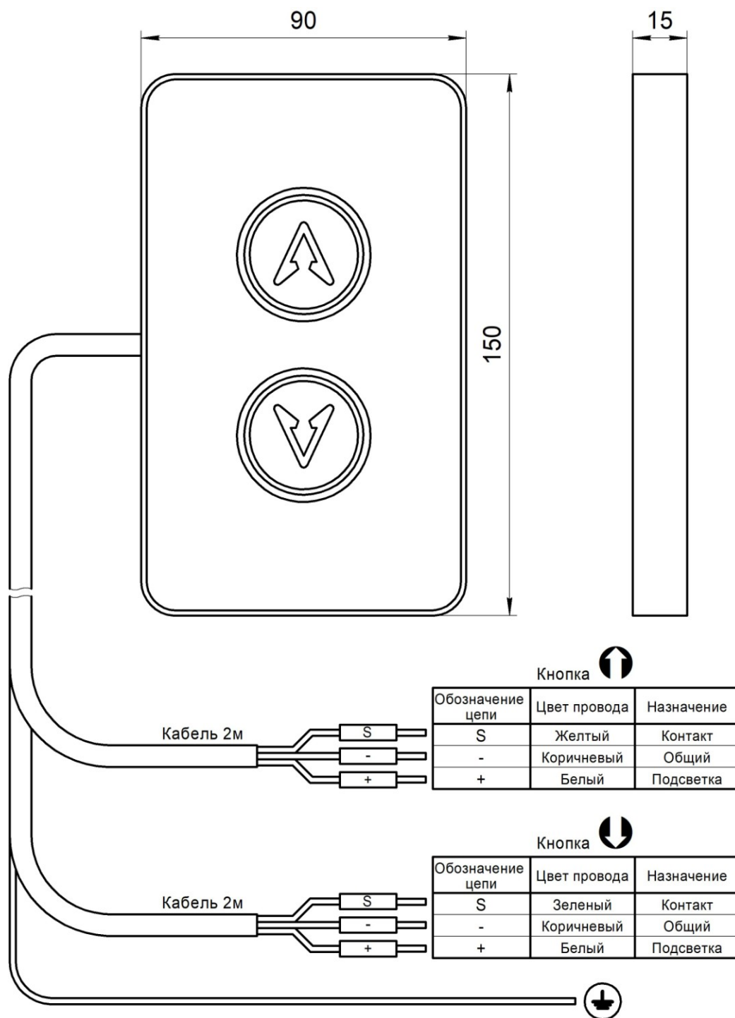
Рис.1 Внешний вид, габаритные и установочные размеры Вызывного поста ОНИКС НШЕК.468381.125-01
